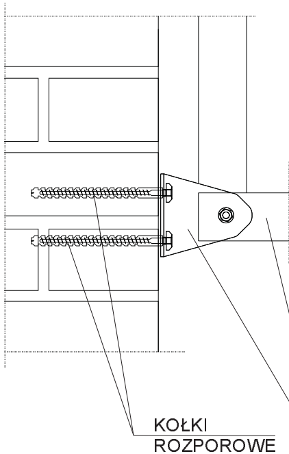
SZCZEGÓŁ "A" ŚCIANA BEZ OCIEPLENIA
