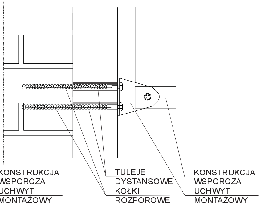
SZCZEGÓŁ "A" ŚCIANA Z OCIEPLENIEM
